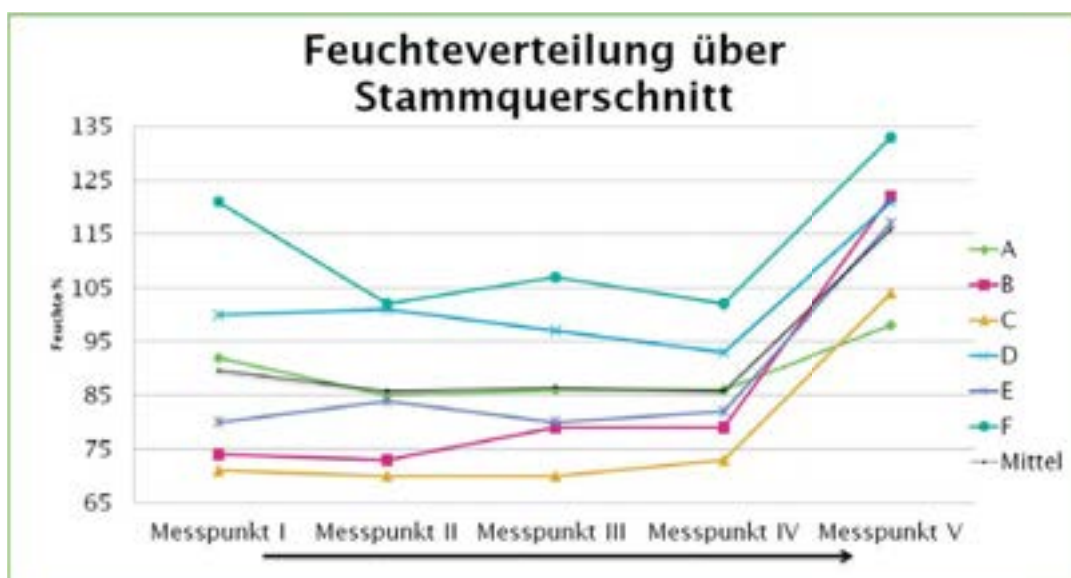
Abbildung 10: Grafische Darstellung der Feuchteverteilung über den Stammquerschnitt aller Probestämme
