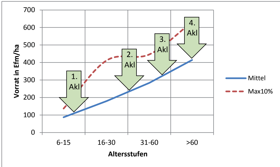
Abbildung 13: Vorräte der Altersbereiche, Übertragung auf die Altersklassen
