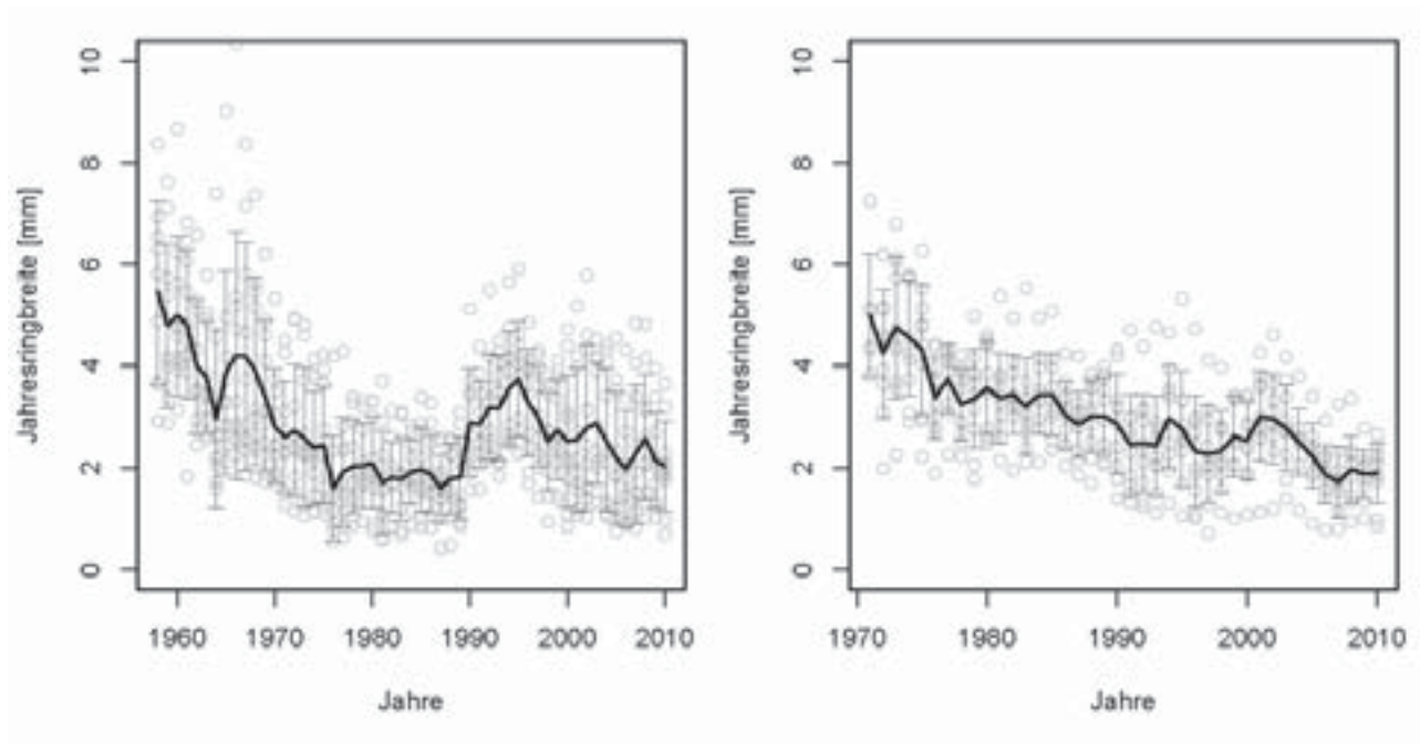
Abbildung 10: Boxplots der Jahresringbreiten der Master Chronologien.
