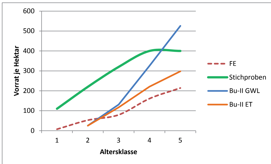
Abbildung 15: Vorräte je Hektar; Vergleich mit Ertragstafel
